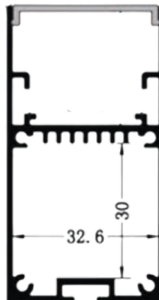
R6635 COD: 7800353
